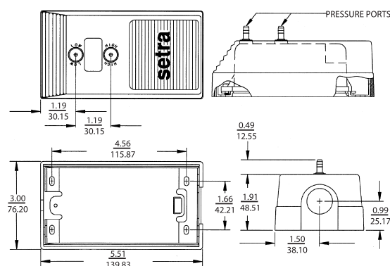
Optional 1/2" Conduit Electrical Enclosure Dimensions
