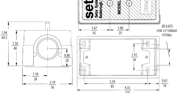
Optional A1 Conduit Electrical Enclosure Dimensions
